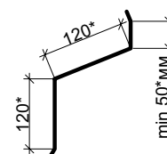
металлический элемент тип 4 (развёртка)
