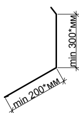
металлический элемент тип 2 (развёртка)
