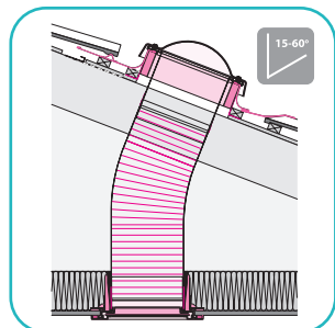
Сечение туннеля с гибкой трубой.
